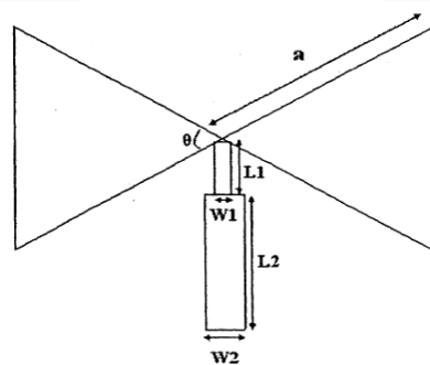
Gambar 2.1 Bentuk antena patch bowtie
