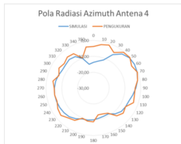
Gambar 4.4 Hasil pengukuran pola radiasi azimuth
