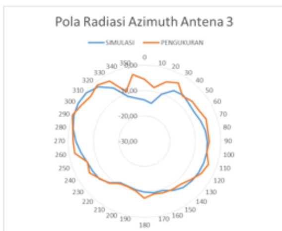
Gambar 4.4 Hasil pengukuran pola radiasi azimuth
