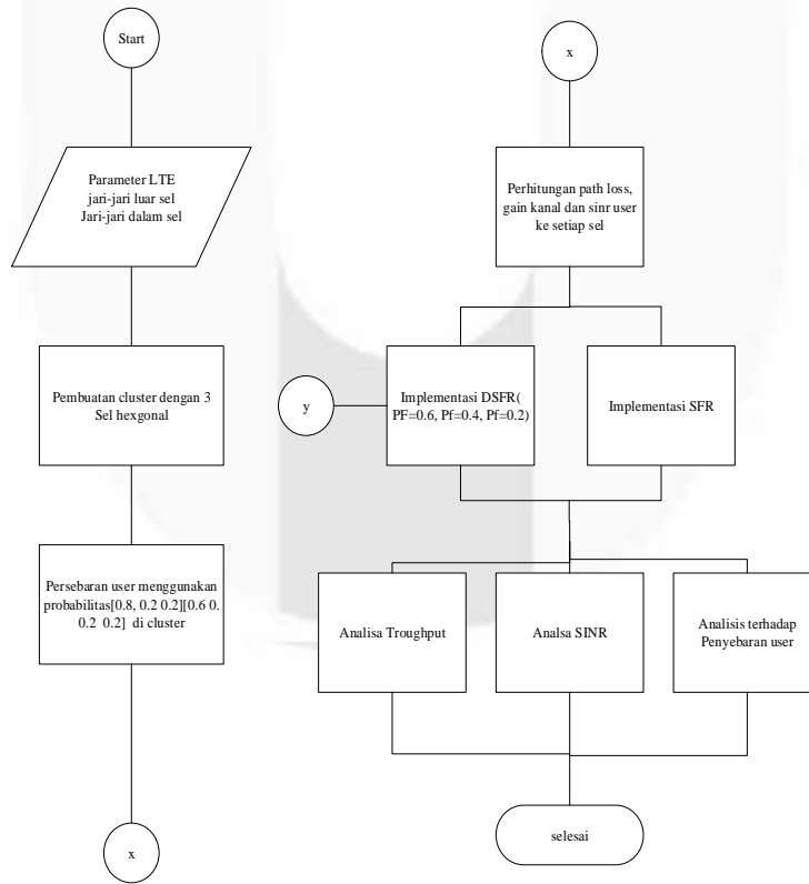
Gambar 3.2 Diagram Alir Skenario Sistem
