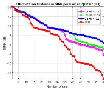
Gambar 3.4 SINR user terhadap urutan user
