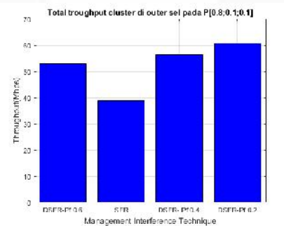
Gambar 3.6 Troughput pada Prob Sel P[sel A;sel B; sel C;]=[0.8;0.1;0.1]
