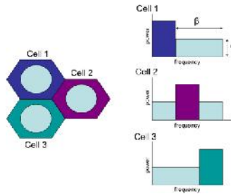
Gambar 2.1 Alokasi Frekuensi dan Daya SFR [9]
