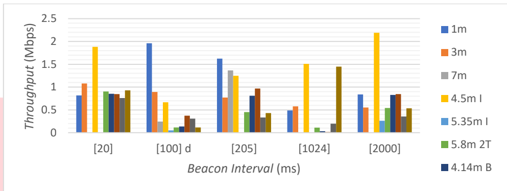
Gambar 3.2 Grafik perubahan nilai beacon interval terhadap nilai throughput
