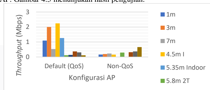
Gambar 3.5 Grafik perbandingan mode QoS dan non-QoS terhadap throughput
