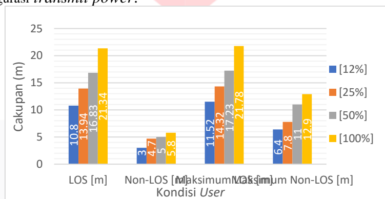
Gambar 3.1 Grafik transmit power dalam persen terhadap jarak user - AP
