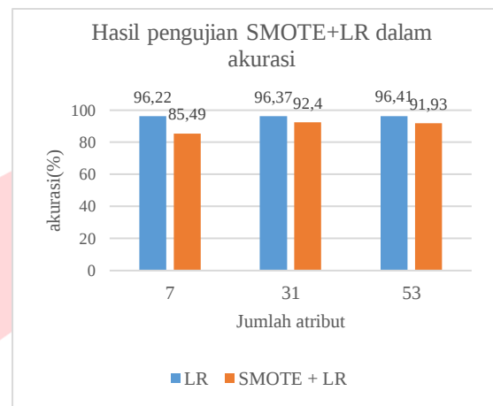
gambar 5 Hasil Pengujian SMOTE+LR dalam akurasi
