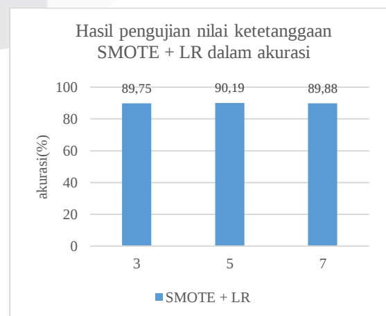
gambar 7 hasil pengujian nilai k dalam akurasi
