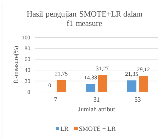
gambar 4 Hasil Pengujian SMOTE+LR dalam f1-measure
