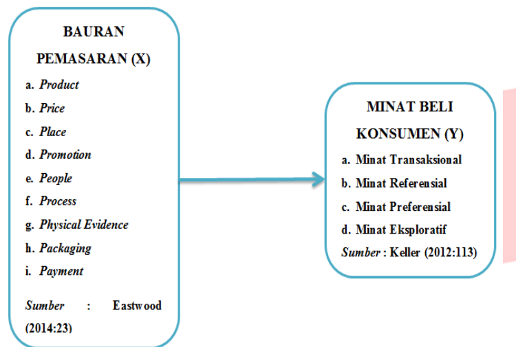
Gambar 2.2 Kerangka Pemikiran
