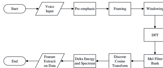
Gambar Error! No text of specified style in document..1 Langkah-langkah MFCC untuk menentukan vektor ciri[9]
