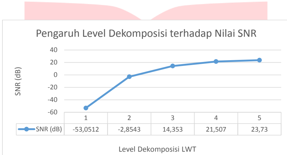
Gambar 4.1 Grafik pengaruh level dekomposisi LWT terhadap SNR
