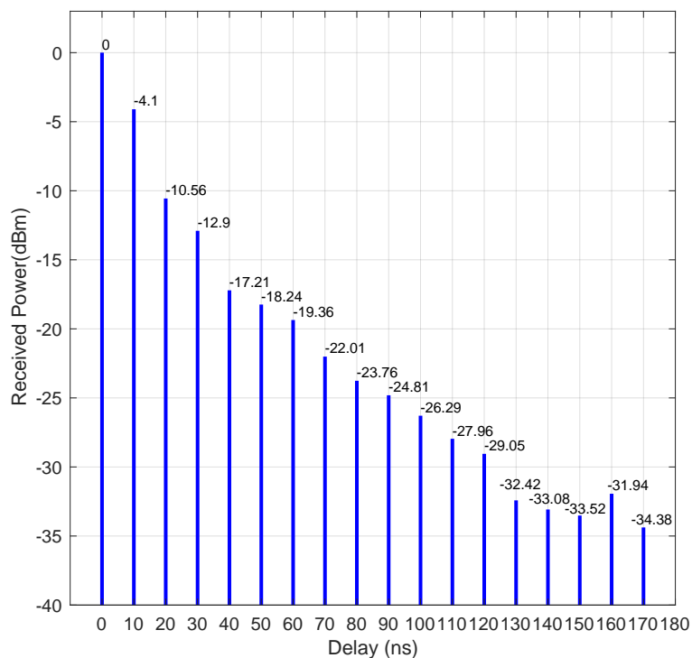
Figure 1: Usulan model kanal 5G Indonesia dengan jarak 200 meter.
