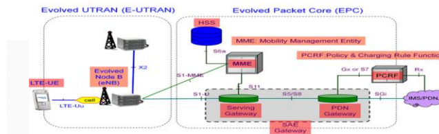
Gambar 2. 1 Arsitektur LTE
