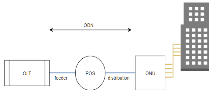
Gambar 2.3 Arsitektur FTTB
