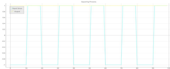
Gambar 3.4 Hasil pengujian dengan memasukkan sinyal square
