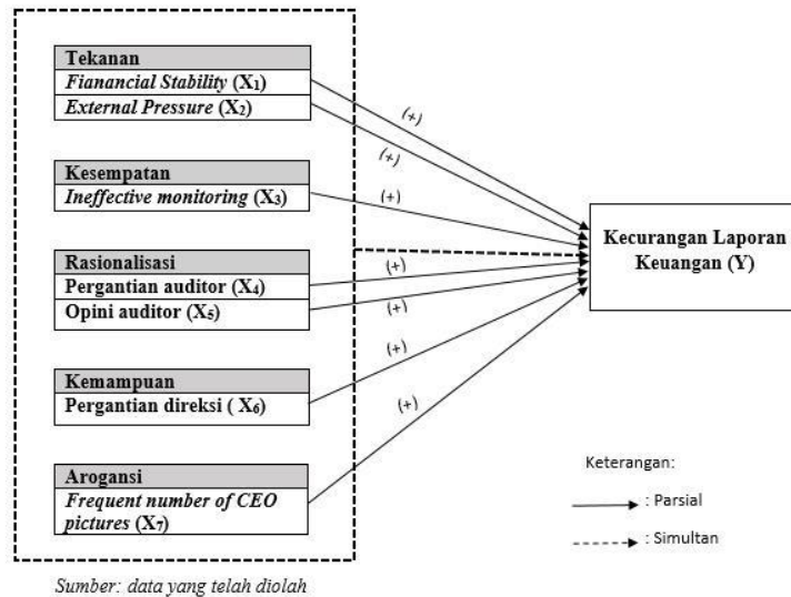
Gambar 2. Kerangka Pemikiran
