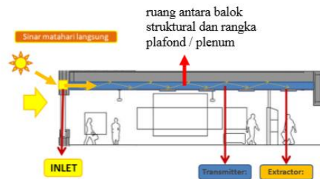
Figur 17. Perletakan inlet dan pipa cahaya horisontal pada potongan gedung tebal
