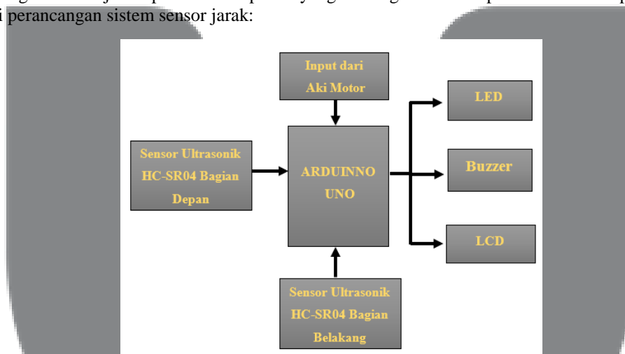
Gambar 3.2 Blok Diagram dari perancangan sistem sensor jarak
