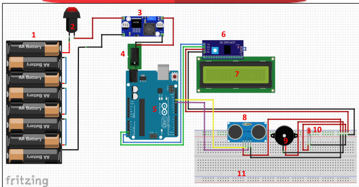
Gambar 3.1 Perancangan sistem pada software fritzing
