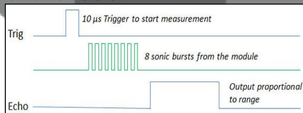
Gambar 2. 3 Visualisasi sinyal dari Sensor HC-SR04 [6]
