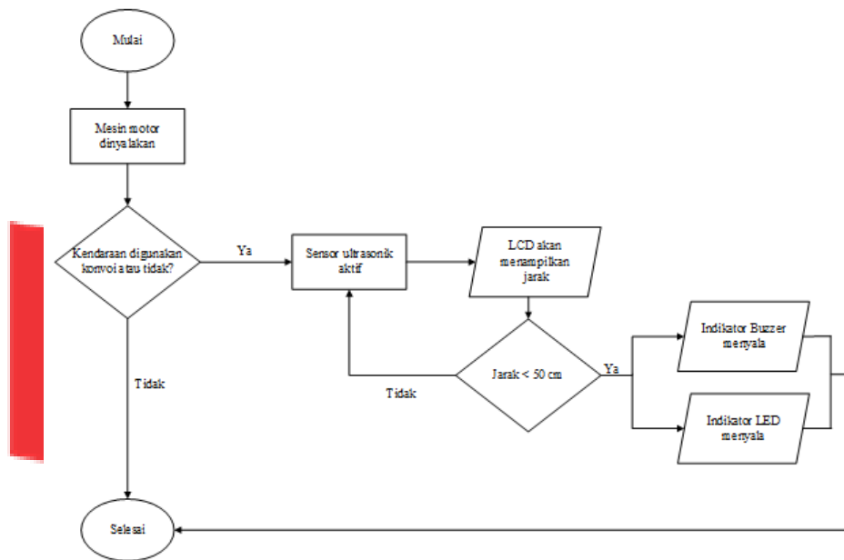
Gambar 3.3 Flow chart sistem pengukuran sensor jarak
