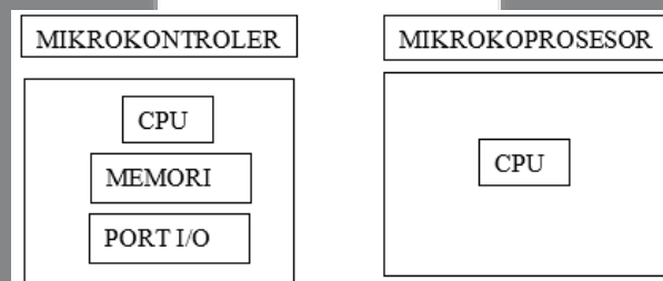
Gambar 2. 1 Perbedaan mikrokontroler dengan mikroprosesor [2] .
