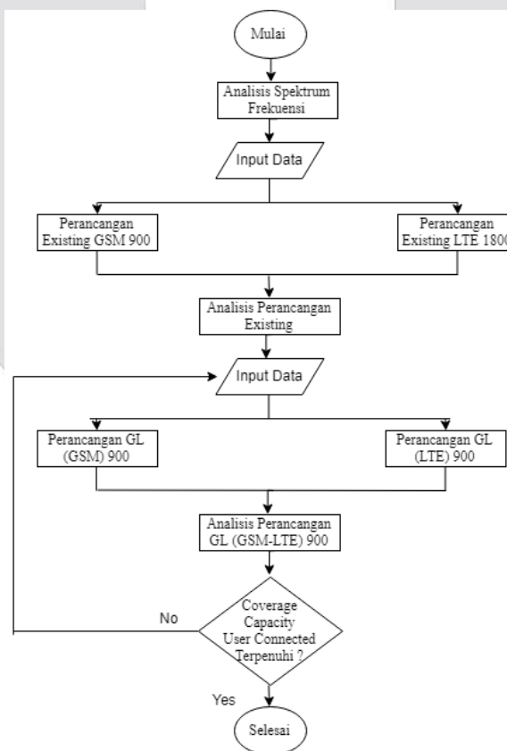
Gambar 3 Diagram Alir Simulasi
