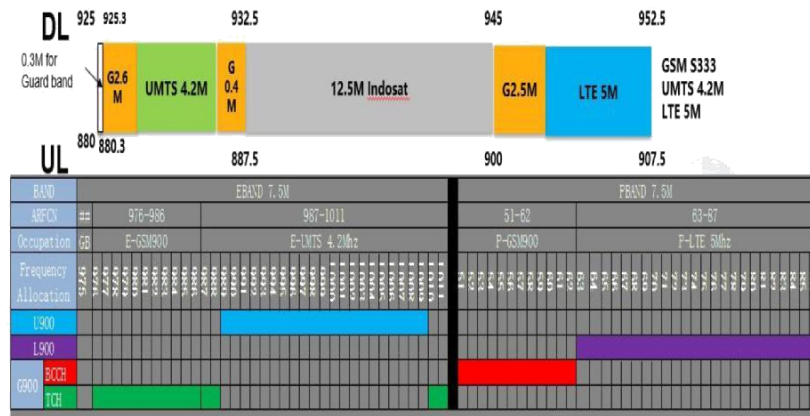
Gambar 1 Alokasi Frekuensi GL Telkomsel [7]
