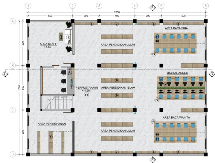
Gambar 7. Layout Perpustakaan
