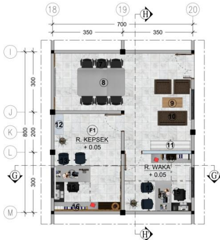
Gambar 5. Layout Ruang Kepala Sekolah & Ruang Wakil Kepala Sekolah
