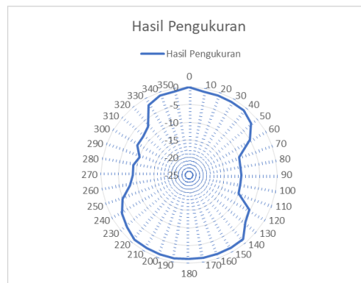
Gambar 9 Pengukuran Polarisasi
