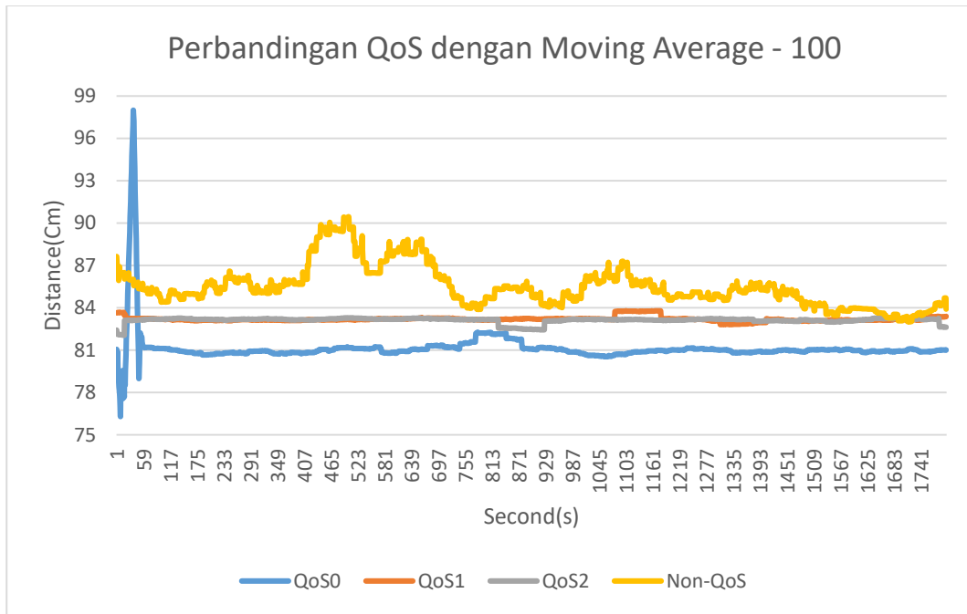
Gambar 8. Data yang diterimakan oleh setiap QoS
