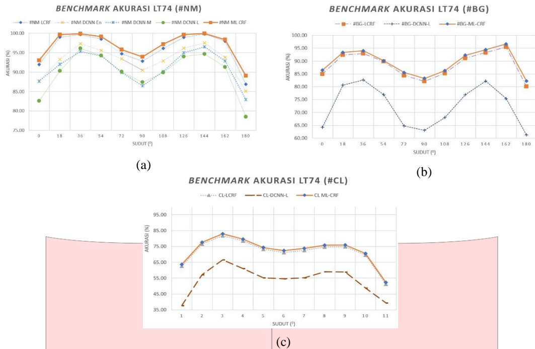
Gambar 2. Hasil benchmark akurasi LT74 (#NM (a), #BG (b), dan #CL (c)).
