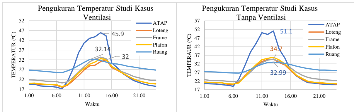
Gambar 3.2 a. Pengukuran Skenario 1 b. Pengukuran skenario 2
