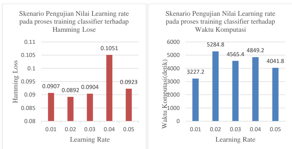
Gambar 4.3 Skenario pengujian dengan nilai learning rate
