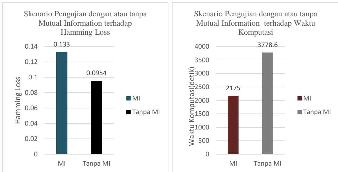
Gambar 4.2 Skenario pengujian dengan atau tanpa Mutual Information terhadap hamming loss
