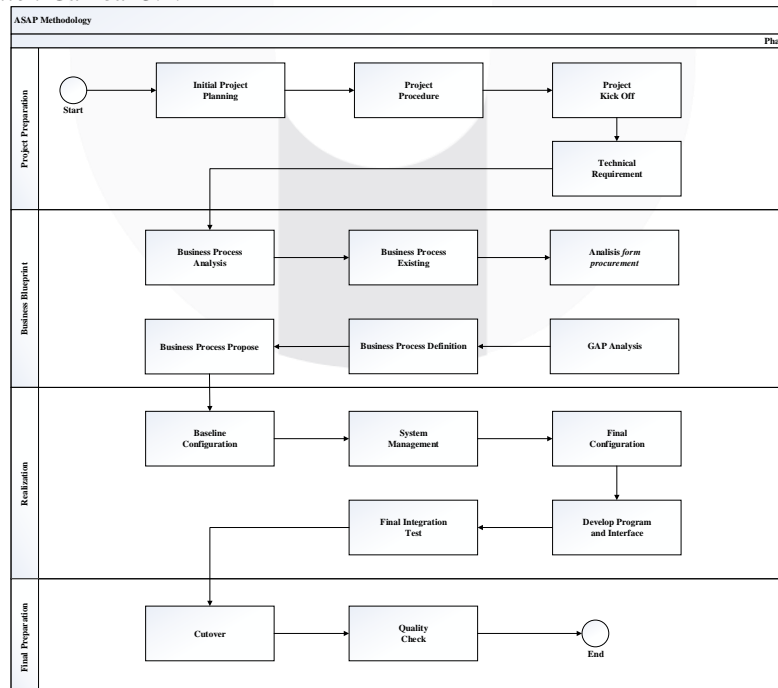
Gambar 3. 2 Sistematika Penelitian
