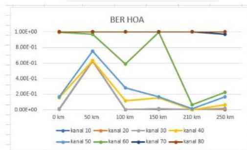
Gambar 10. Nilai BER
