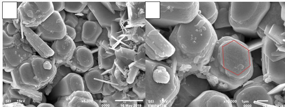
Gambar 4.4 Hasil karakterisasi morfologi dengan SEM sampel nanas madu kalsinasi 800°C (1) berbentuk seperti heksagonal. a) Perbesaran 5000 kali, b) Perbesaran 10.000 kali.
