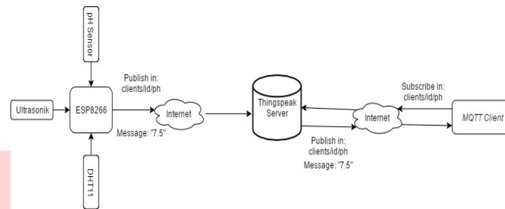
Gambar 3 Perancangan IOT
