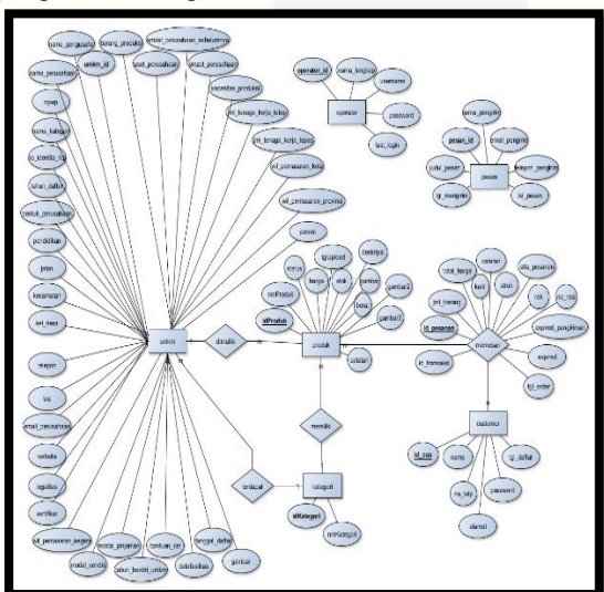
Gambar 3 - 8. ERD
