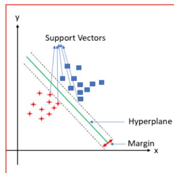
Gambar 1. Struktur SVM [8]
