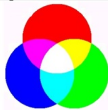
Gambar 2. 3 Citra RGB
