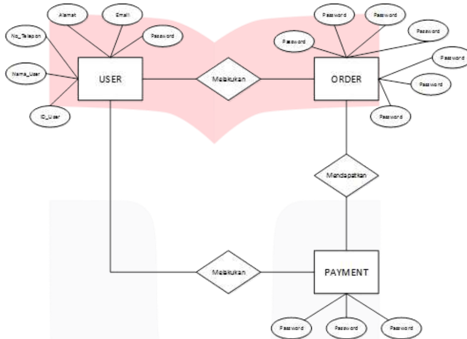
Gambar 4 ERD
