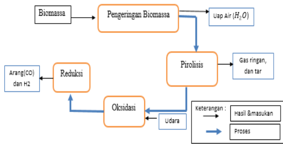
Gambar 2. Tahapan gasifikasi;
