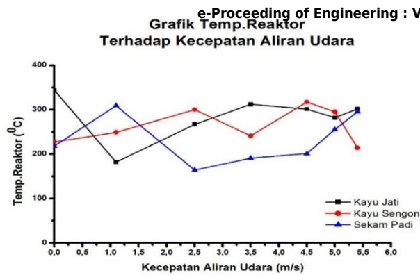
Gambar 12. Grafik Temp.Reaktor pada kompor gasifikasi biomassa ditiap variasi jenis biomassa dengan kecepatan aliran udara,
