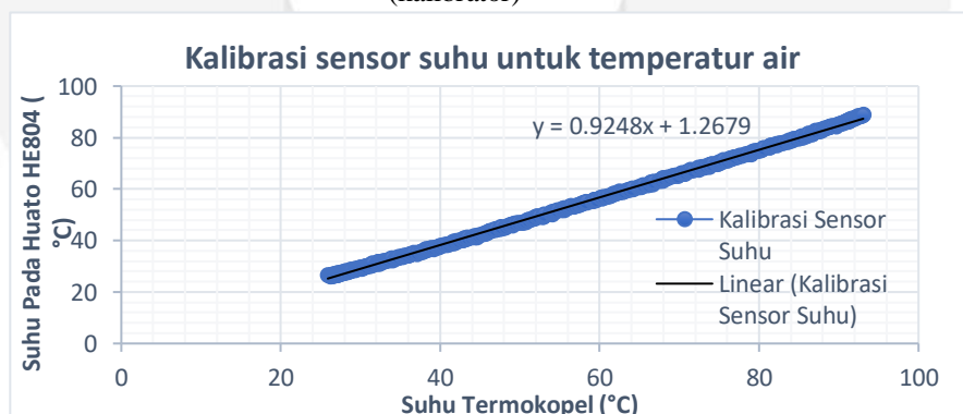
Gambar 7. Kurva kalibrasi sensor suhu untuk temperatur air yang digunakan terhadap instrumen standar (kalibrator)
