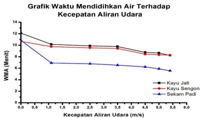
Gambar 11. Grafik waktu mendidihkan air pada kompor gasifikasi biomassa ditiap variasi jenis biomassa dengan kecepatan aliran udara
