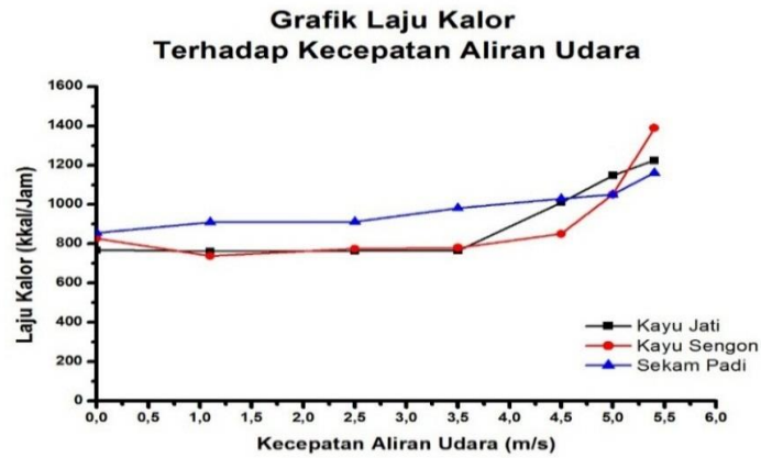
Gambar 10. Grafik Laju Kalor kompor gasifikasi biomassa ditiap variasi jenis biomassa dengan kecepatan aliran udara;
