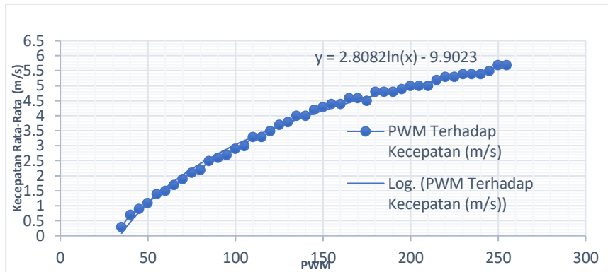
Gambar 8. Kurva karakterisasi kecepatan aliran udara kipas terhadap nilai PWM yang diberikan.
