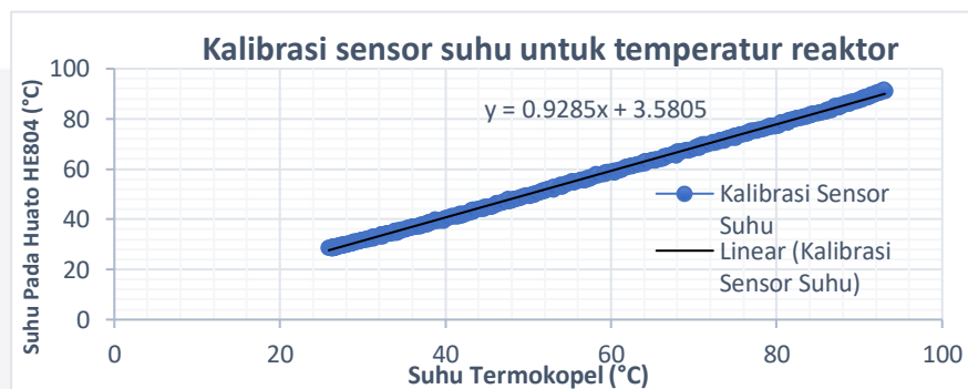
Gambar 6 Kurva kalibrasi sensor suhu untuk temperatur reaktor yang digunakan terhadap instrumen standar (kalibrator)
