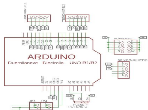
Gambar 5. Sistem Elektrik
