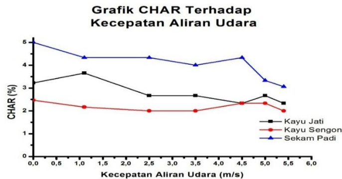
Gambar 13. Grafik persentase char yang dihasilkan pada kompor gasifikasi biomassa ditiap variasi jenis biomassa dengan kecepatan aliran udara.
