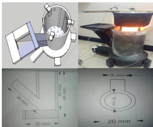
Gambar 4. Rancangan Kompor
