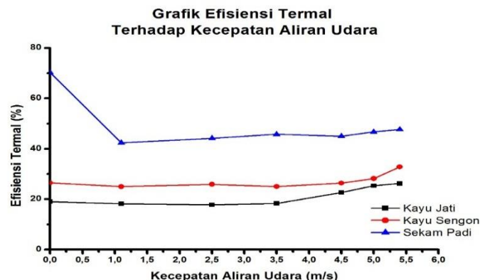
Gambar 14. Grafik efisiensi termal pada kompor gasifikasi biomassa ditiap variasi jenis biomassa dengan kecepatan aliran udara
