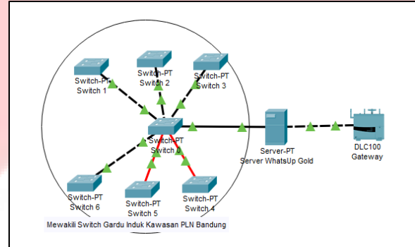
Gambar 2.1. Gambar Sistem Saat Ini
