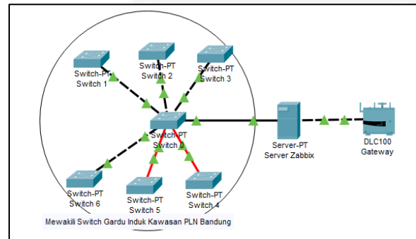
Gambar 3.2 Gambaran Sistem Usulan
