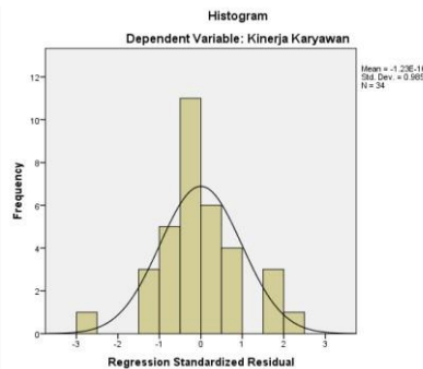
Gambar 2 Grafik Histogram
