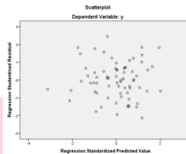
Gambar 4 Grafik Scatterplot
