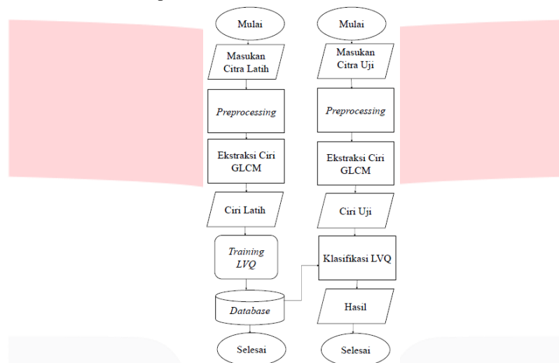
Gambar 6 Flowchart sistem pelatihan dan pengujian
