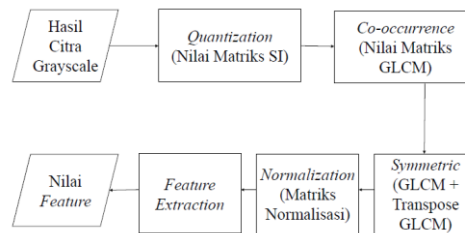
Gambar 5 Diagram Alir Ekstraksi Ciri GLCM.
