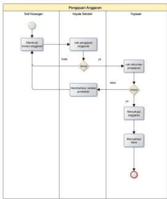
Gambar 3-1. Proses Berjalan Pengajuan Anggaran
