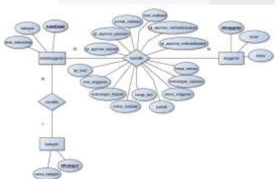
Gambar 3-6. Usecase Diagram
