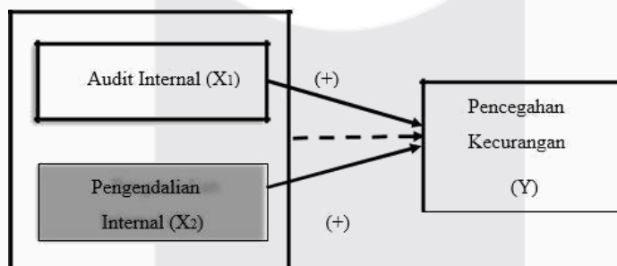
Gambar 2.1 Kerangka Pemikiran
