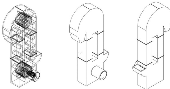
Gambar 6. Desain Alat Bantu Terpilih
