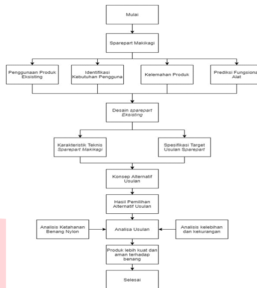
Gambar 5. Metodologi Penelitian
