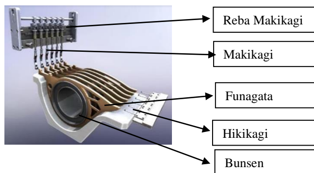
Gambar 6. Dekomposisi Produk
