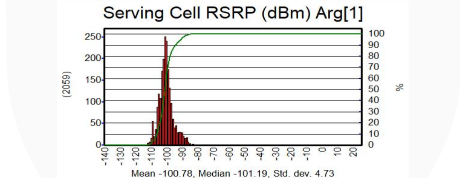
Gambar 8 Grafik Hasil Walktest RSRP pada area lantai 3 check-in bandara
