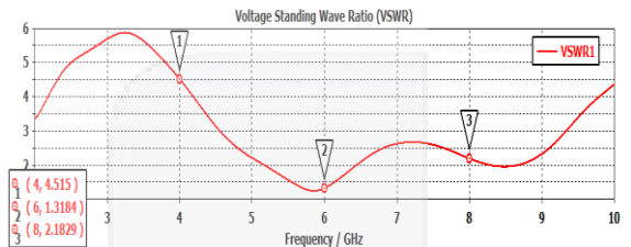
Gambar 3.5 Hasil VSWR setelah optimasi
