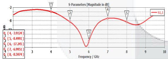
Gambar 3.4 Hasil return loss simulasi awal
