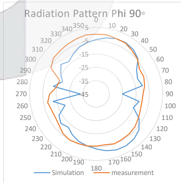
Gambar 4.3 Hasil polaradiasi berdasarkan elevasi
