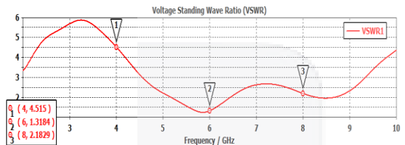
Gambar 3.3 Hasil VSWR simulasi awal
