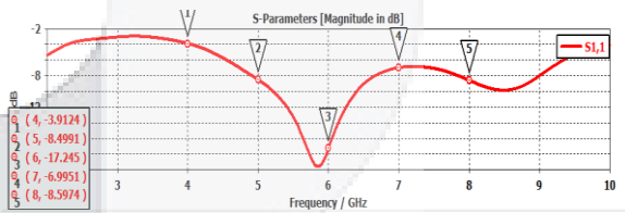
Gambar 3.6 Hasil return loss setelah optimasi
