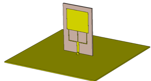
Gambar 3.2 Desain antenna
