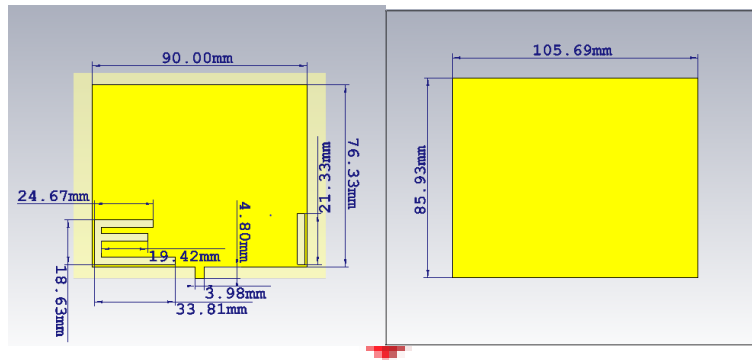
Gambar 1. Rancangan awal antenna mikrostrip
