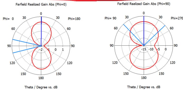
Gambar 7. Pola radiasi pada frekuensi 0,95 GHz
