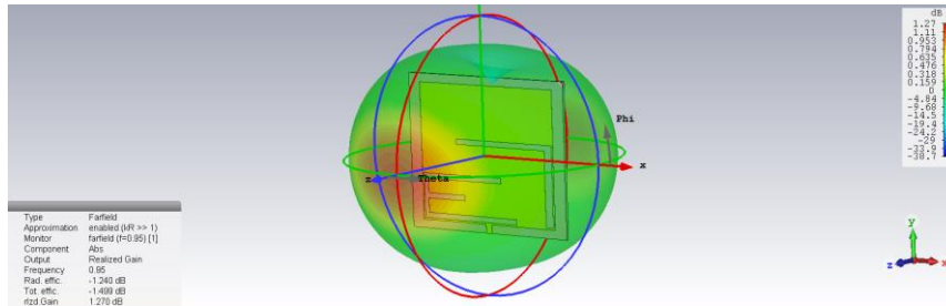
Gambar 6. Medan jauh pada frekuensi 0,95 GHz
