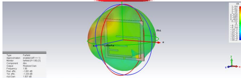
Gambar 10. Medan jauh pada frekuensi 1,85 Ghz
