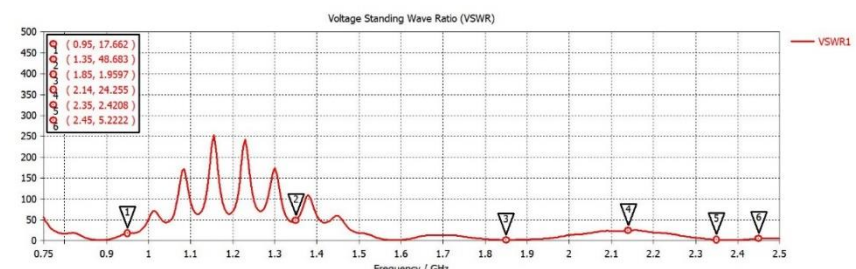
Gambar 2. Grafik VSWR
