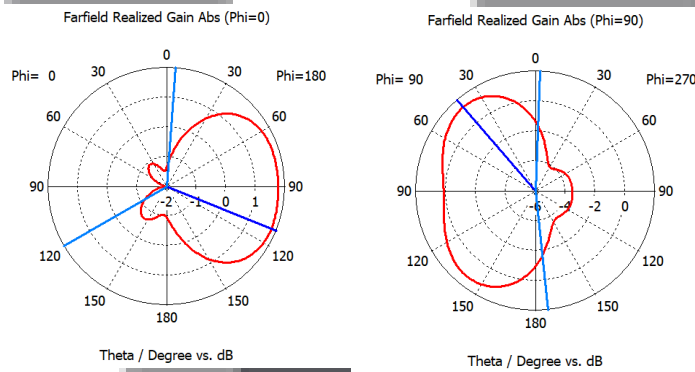
Gambar 11. Pola radiasi pada frekuensi 1,85 GHz
