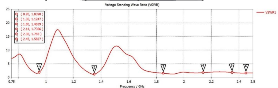
Gambar 5. Grafik VSWR
