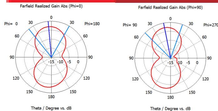
Gambar 17. Pola radiasi pada frekuensi 2,45 GHz
