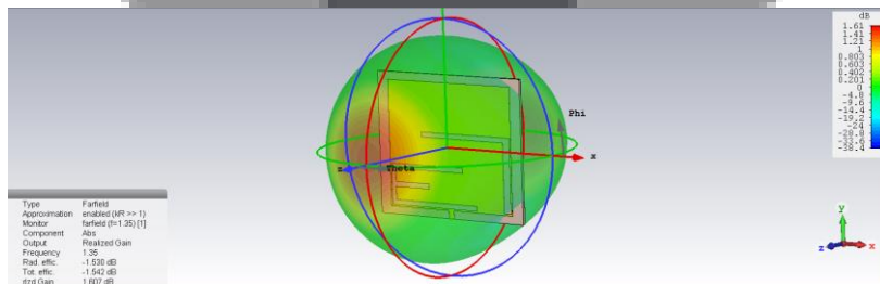
Gambar 8. Medan jauh pada frekuensi 1,35 GHz
