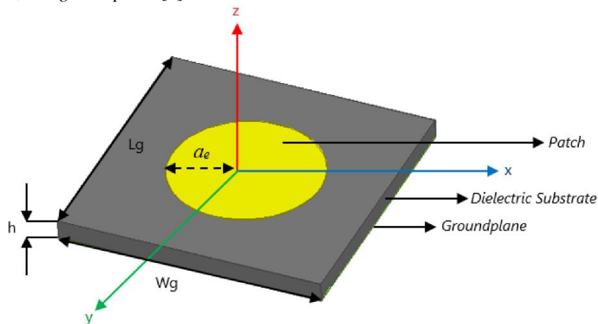
Gambar 1 Antena
