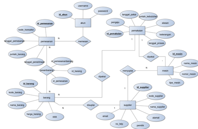
Gambar 2-3 ERD
