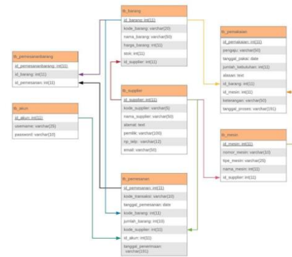
Gambar 2-4 Skema Relasi
