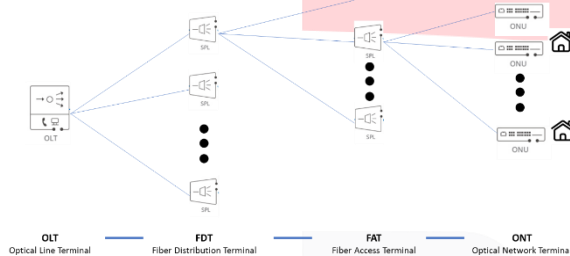
Gambar 3 Teknologi GPON
