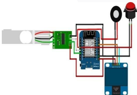
Gambar 5. Desain Perangkaian Alat
