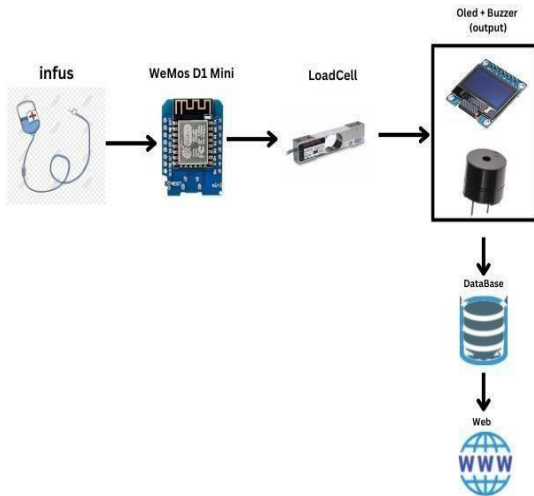
Gambar 2. Desain Sistem Alat
