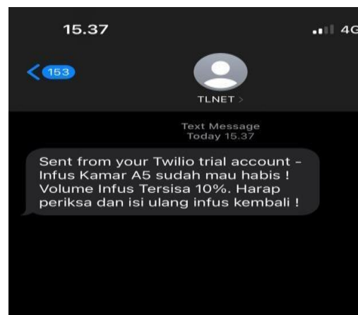
Gambar 7. Notifikasi SMS
