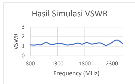
Gambar 10. Hasil VSWR
