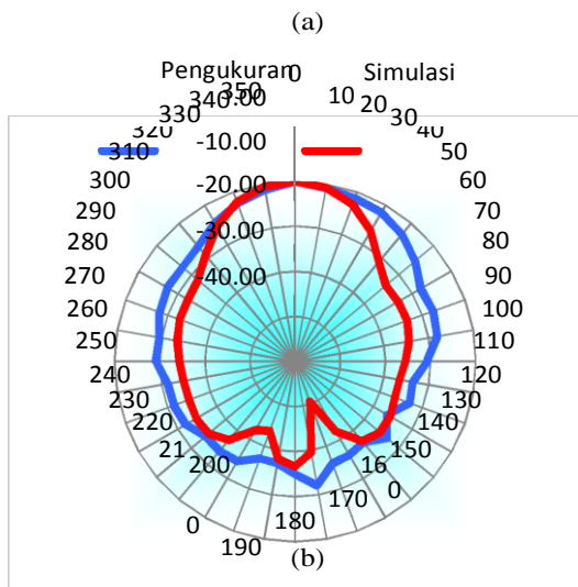
Gambar 10 Hasil Pengukuran Pola Radiasi (a) Azimuth (b) elevasi
