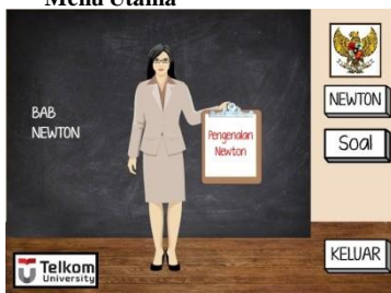
Gambar 3.1 Menu Utama
