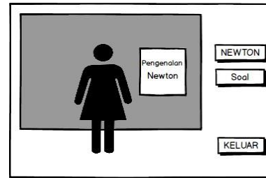
Gambar 1.4 Menu Utama
