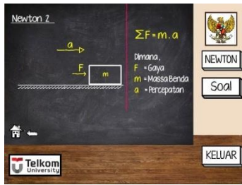
Gambar 3.6 Materi Newton 2
