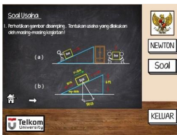
Gambar 3.14 Soal Usaha
