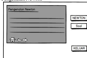
Gambar 1.5 Pengenalan Newton
