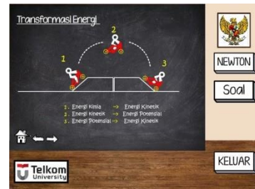
Gambar 3.11 Transformasi Energi
