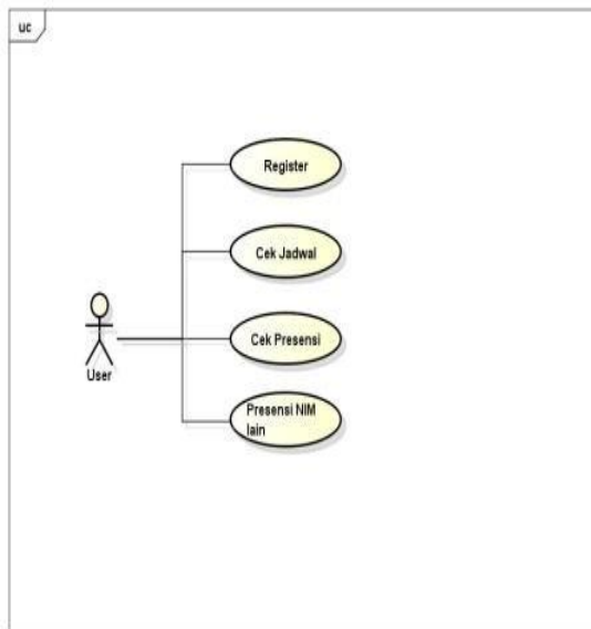
Gambar 3.3 use case diagram aplikasi
