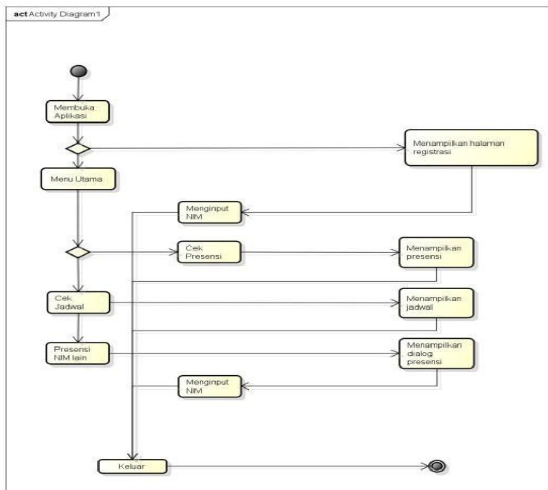
Gambar 3.2 activity diagram aplikasi
