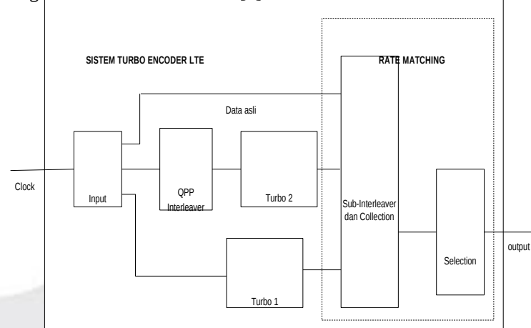
Gambar 4. Struktur Turbo Encoder dispesifikasikan oleh 3GPP diadaptasi dari [3]
