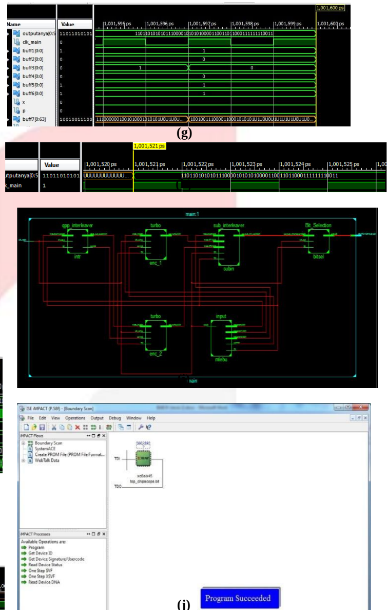
Gambar 6 Hasil Simulasi pada ISim (a) Input QPP Interleaver (b) Output QPP Interleaver (c) Output Turbo1 (d) Output Turbo2 (e)(f)(g) Output Sub-Interleaver (h) Hasil Turbo Encoder sebelum dimodulasikan (i) Hasil sintesis (j) Program sukses ditanamkan di FPGA
