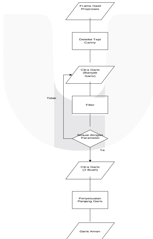
Gambar 3.5 Diagram alir pembentukan garis area aman menggunakan deteksi tepi Canny
